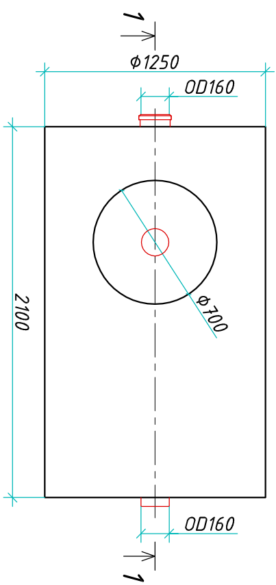
Вид сверху
