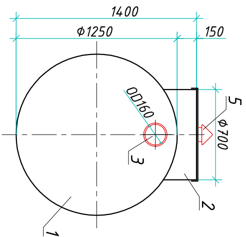
Вид А
