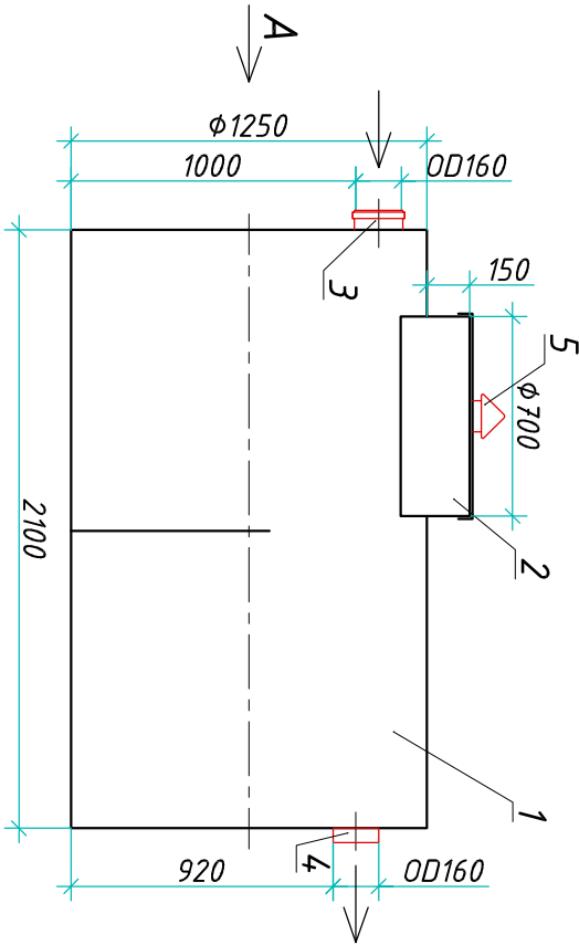
Разрез 1-1
